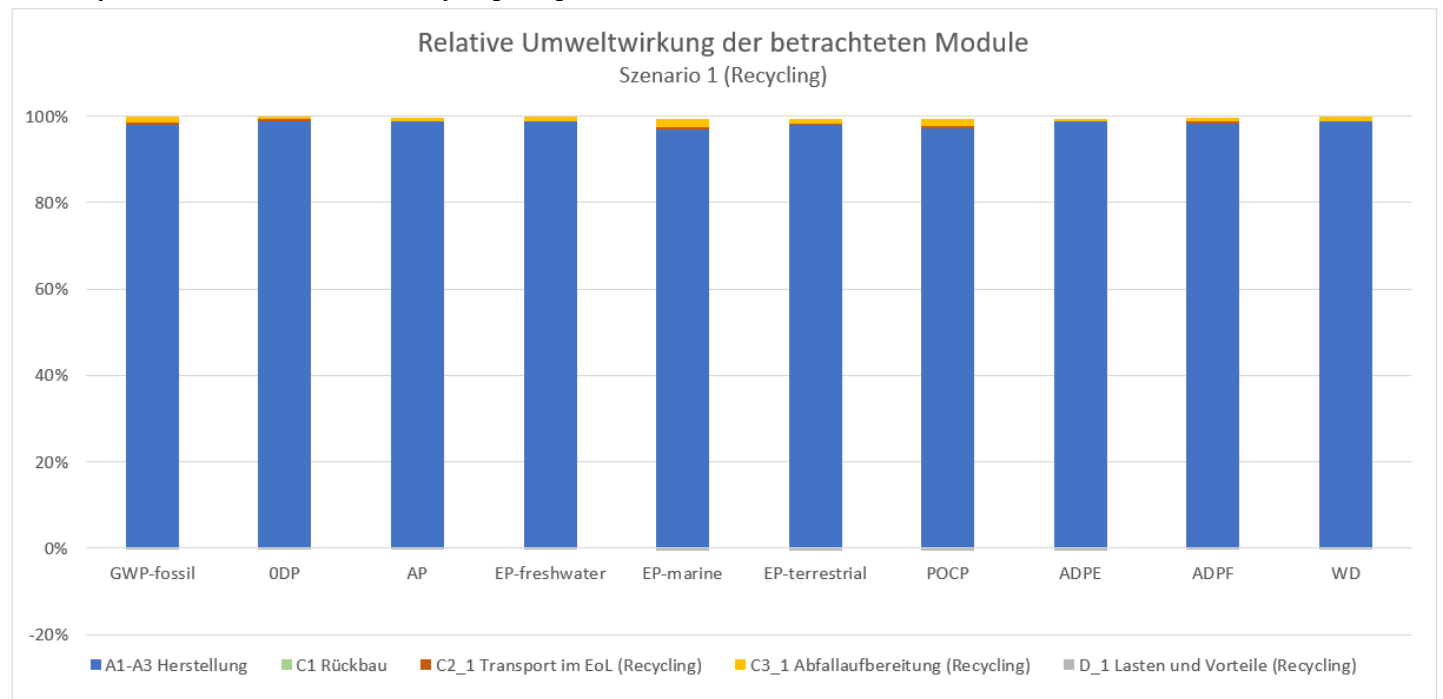
Abbildung 1: Relative Beiträge der einzelnen Abschnitte des Lebenszyklus von Verbund-Sicherheitsglas zu den Indikatoren der Wirkungsabschätzung (EoL-Szenario: Recycling); Module A1–C4 = 100 %
